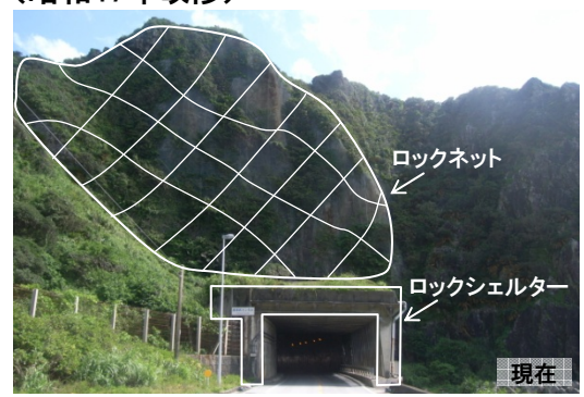
②2代目トンネル:座津武トンネル (昭和47年改修)
