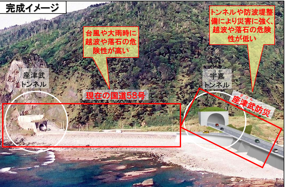
▲図 座津武防災の完成イメージ
